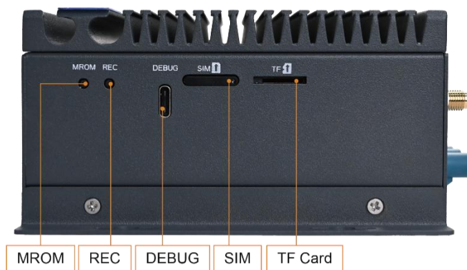
图 2-3 MRC-P5760 机器人控制器侧面接口标注图
