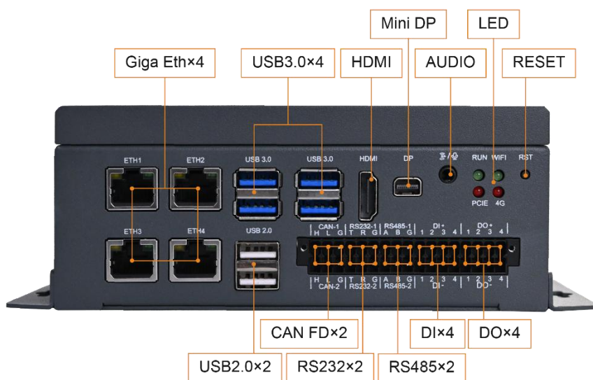
图 2-1 MRC-P5760 机器人控制器正面接口标注图
