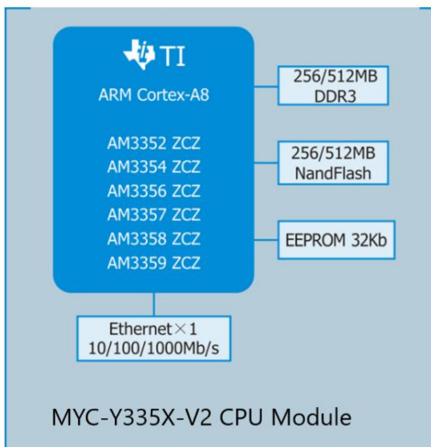
图 2-2 核心板板载资源配置
